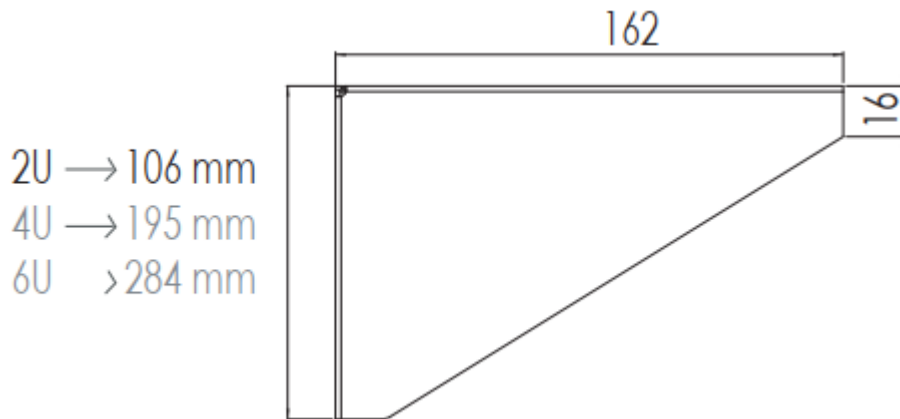
VUE COTE
