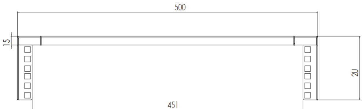
VUE COTE
