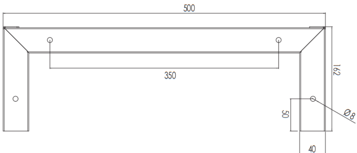
VUE ARRIERE
