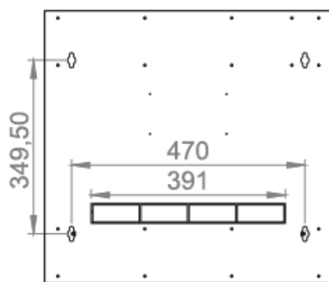
VUE ARRIÈRE
