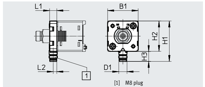
[1] M8 plug
