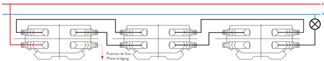
Conmutador cruce / Intermediate switch 10000251-039
