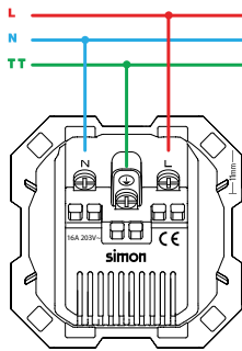
Base de enchufe IO / Simon IO Socket 10002432-039
