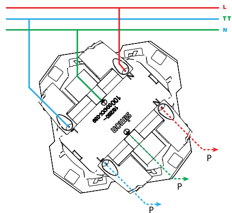
Base bipolar con toma de tierra schuko/ German socket, 1-click terminal connection 10000432-039
