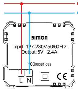
Cargador 2x USB / 2x-port USB charger 1000381-039
