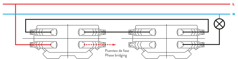
Conmutador / 2-way switch 10000201-039
