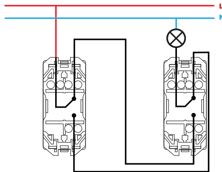
Conmutador / 2-way switch 20000201-XXX
