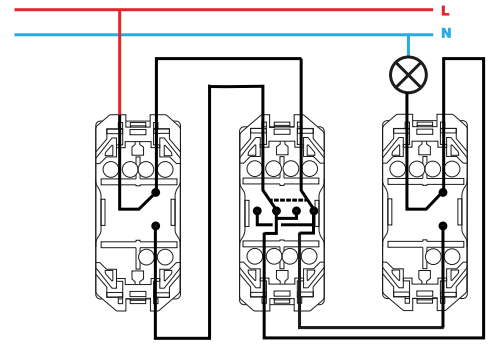
Conmutador cruce / Intermediate switch 20000251-XXX
