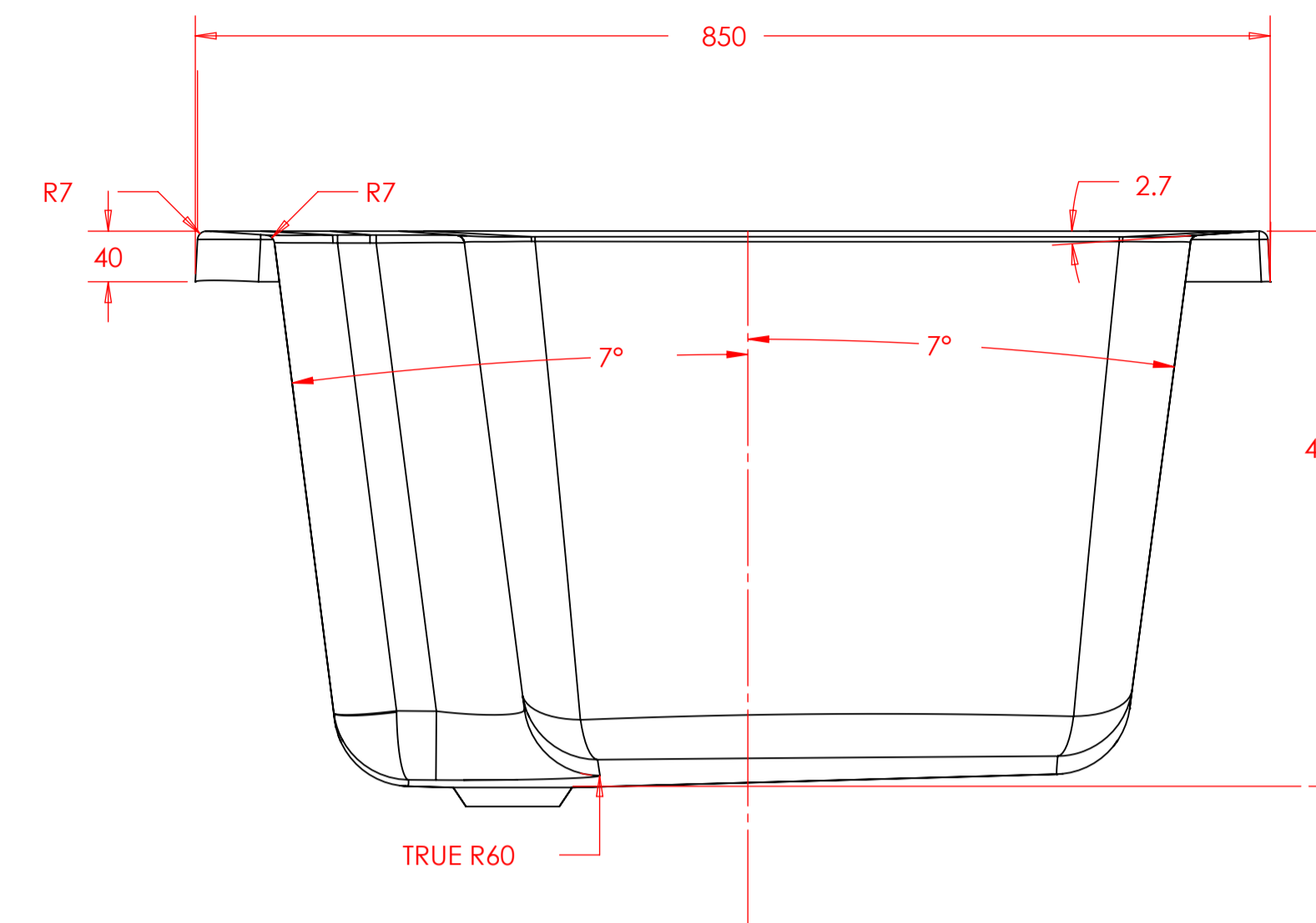
SECTION A-A SCALE 1 : 5
