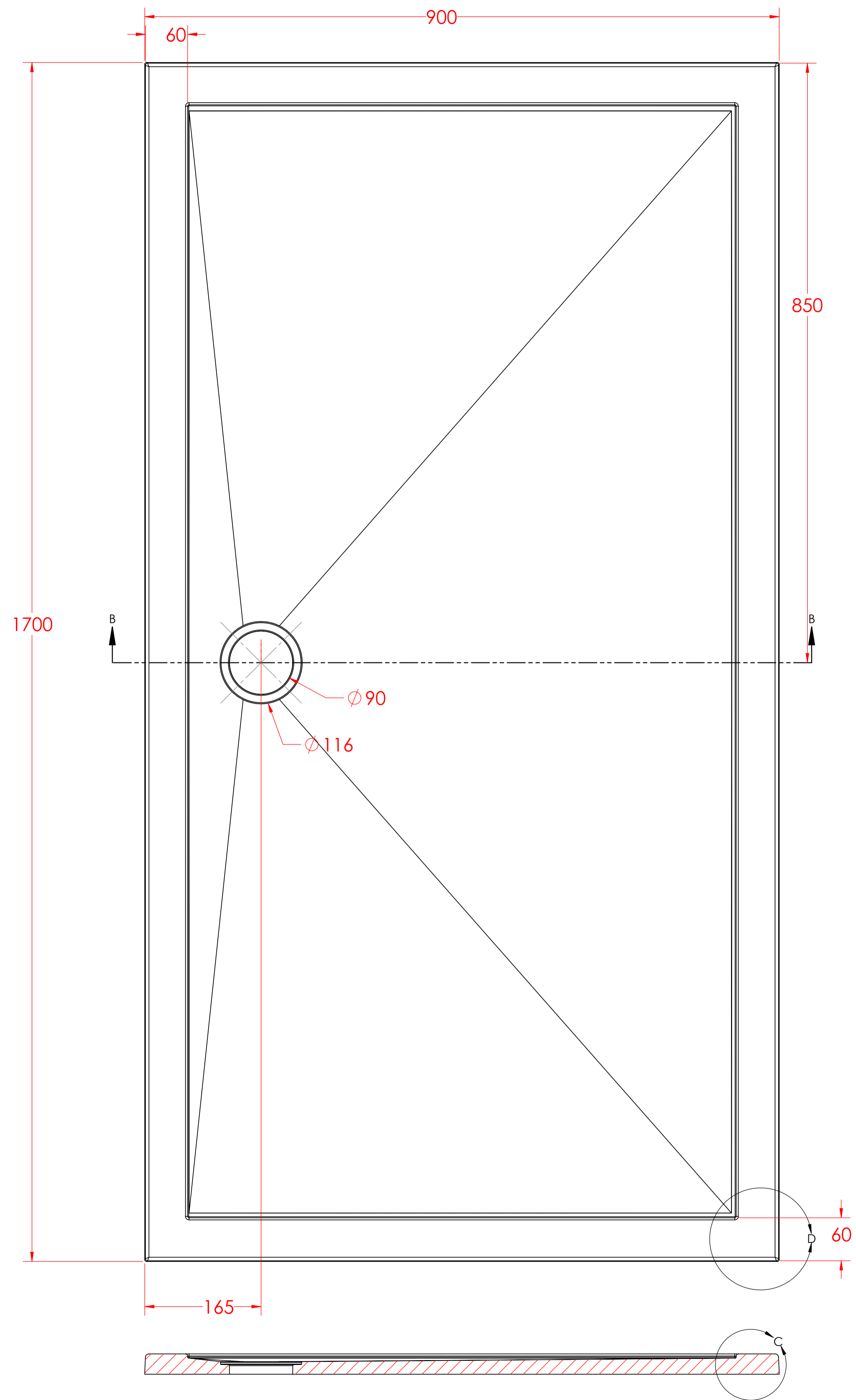
SECTION B-B SCALE 1 : 4
