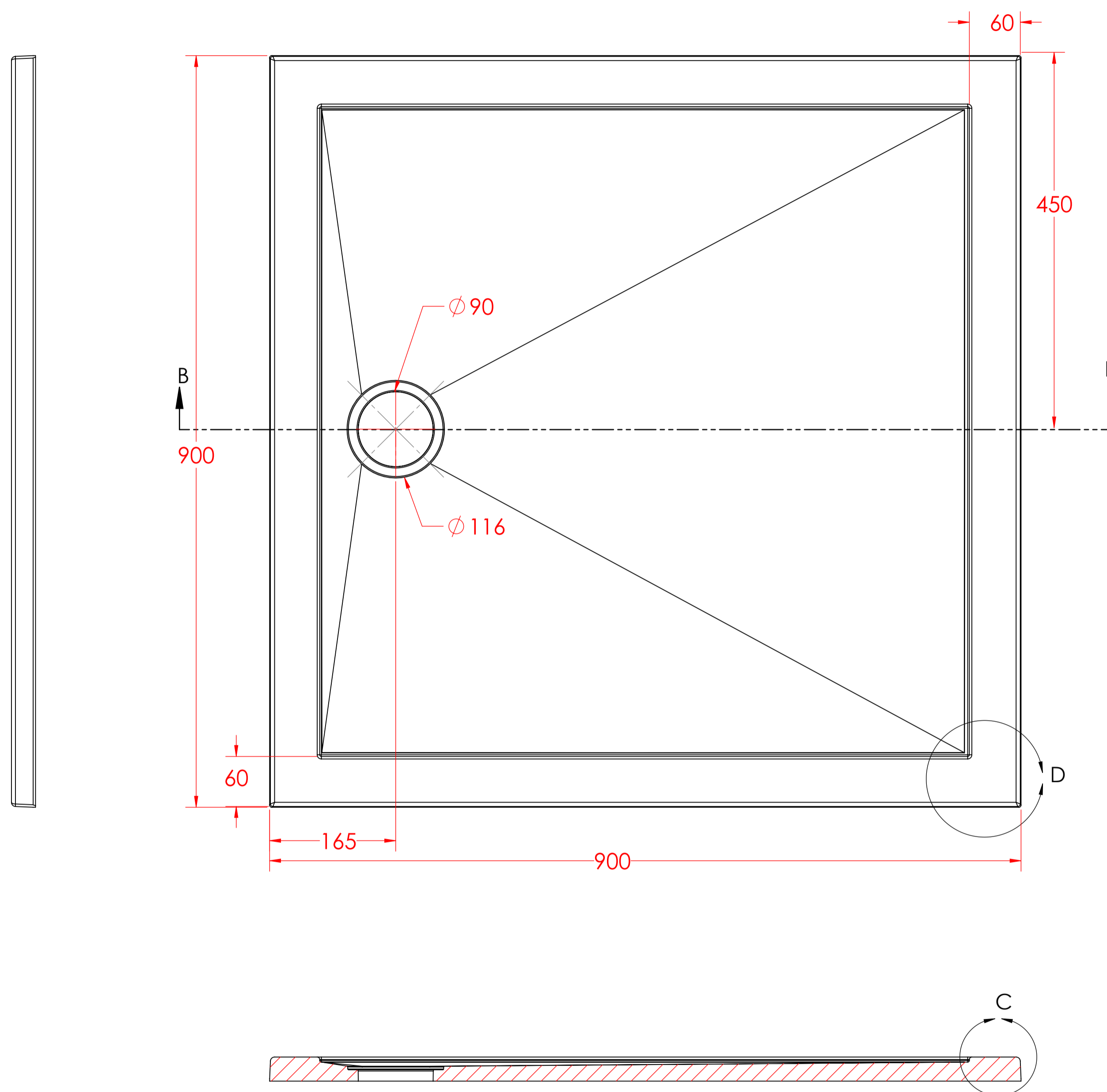
SECTION B-B SCALE 1 : 4
