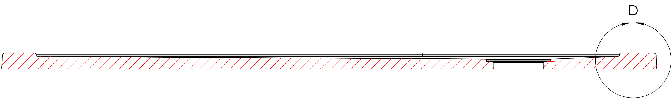
SECTION B-B SCALE 1 : 4
