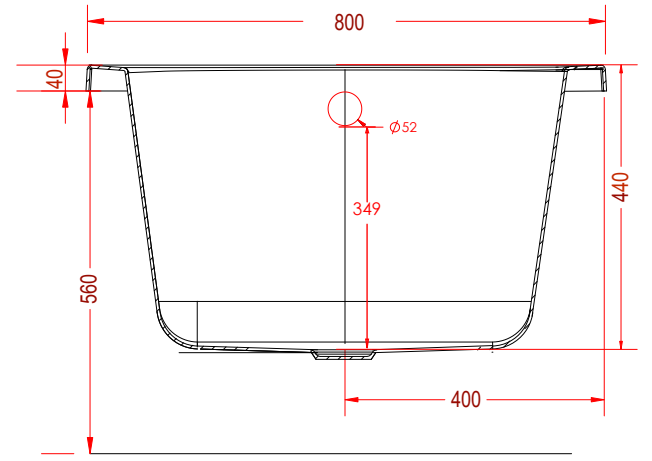
SECTION A-A SCALE 1:4
