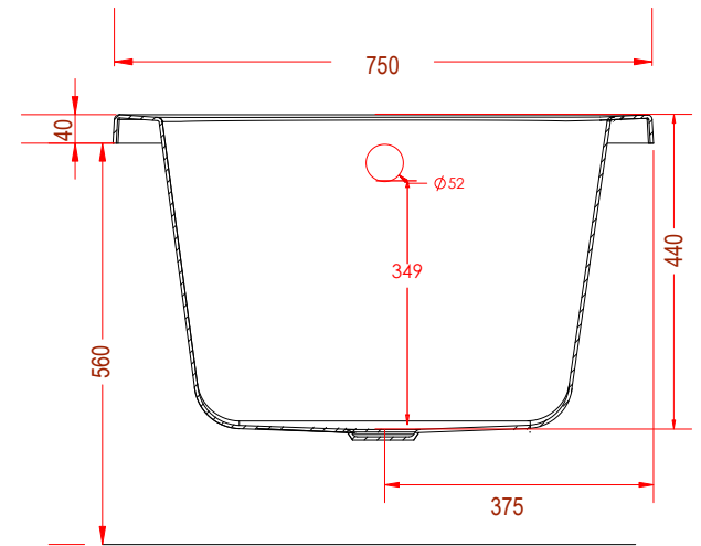
SECTION A-A SCALE 1 : 4
