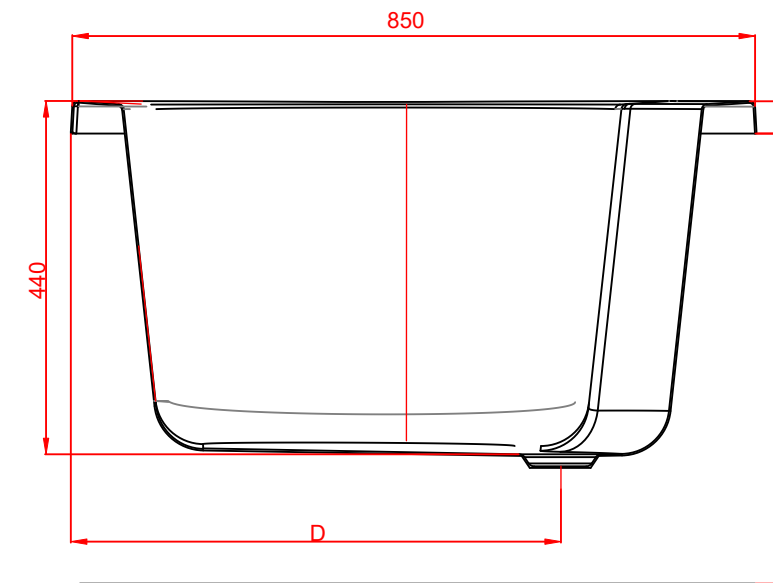
SECTION A-A SCALE 1:4
