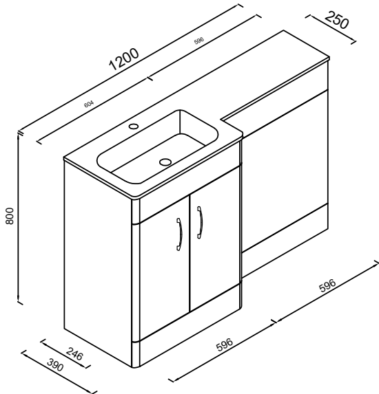
Chaddesley 600+600(LH)
