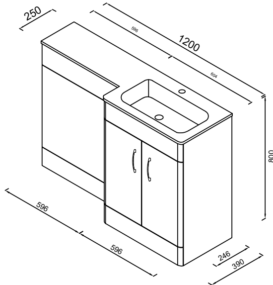
Chaddesley 600+600(RH)
