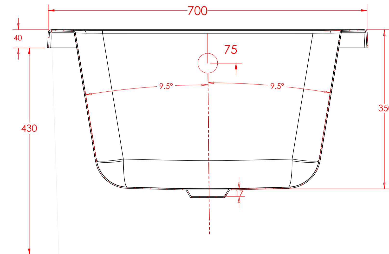
SECTION A-A SCALE 1 : 4
