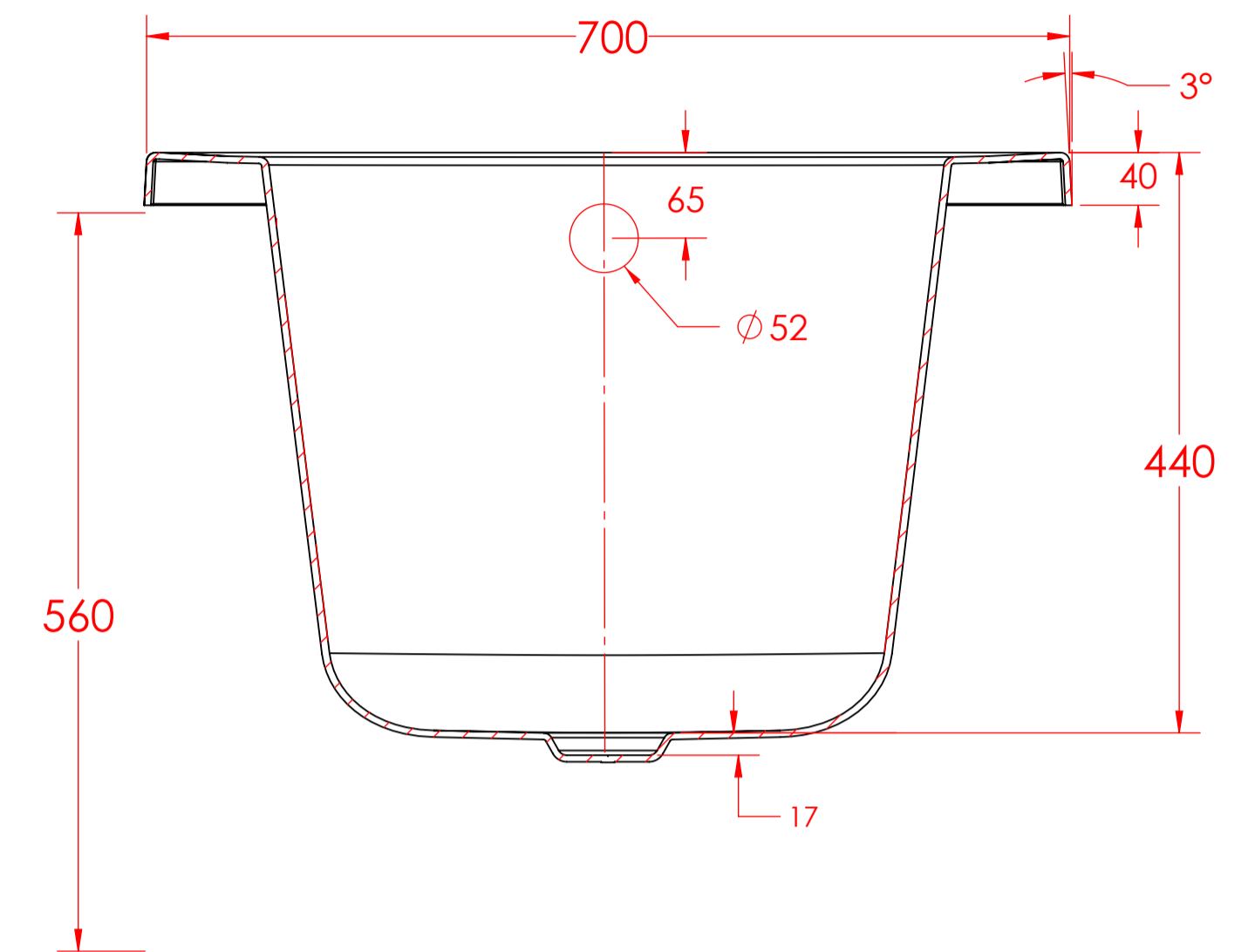
SECTION A-A
