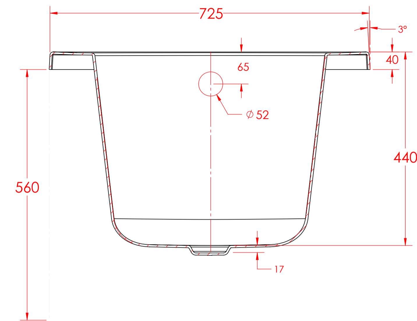
SECTION A-A
