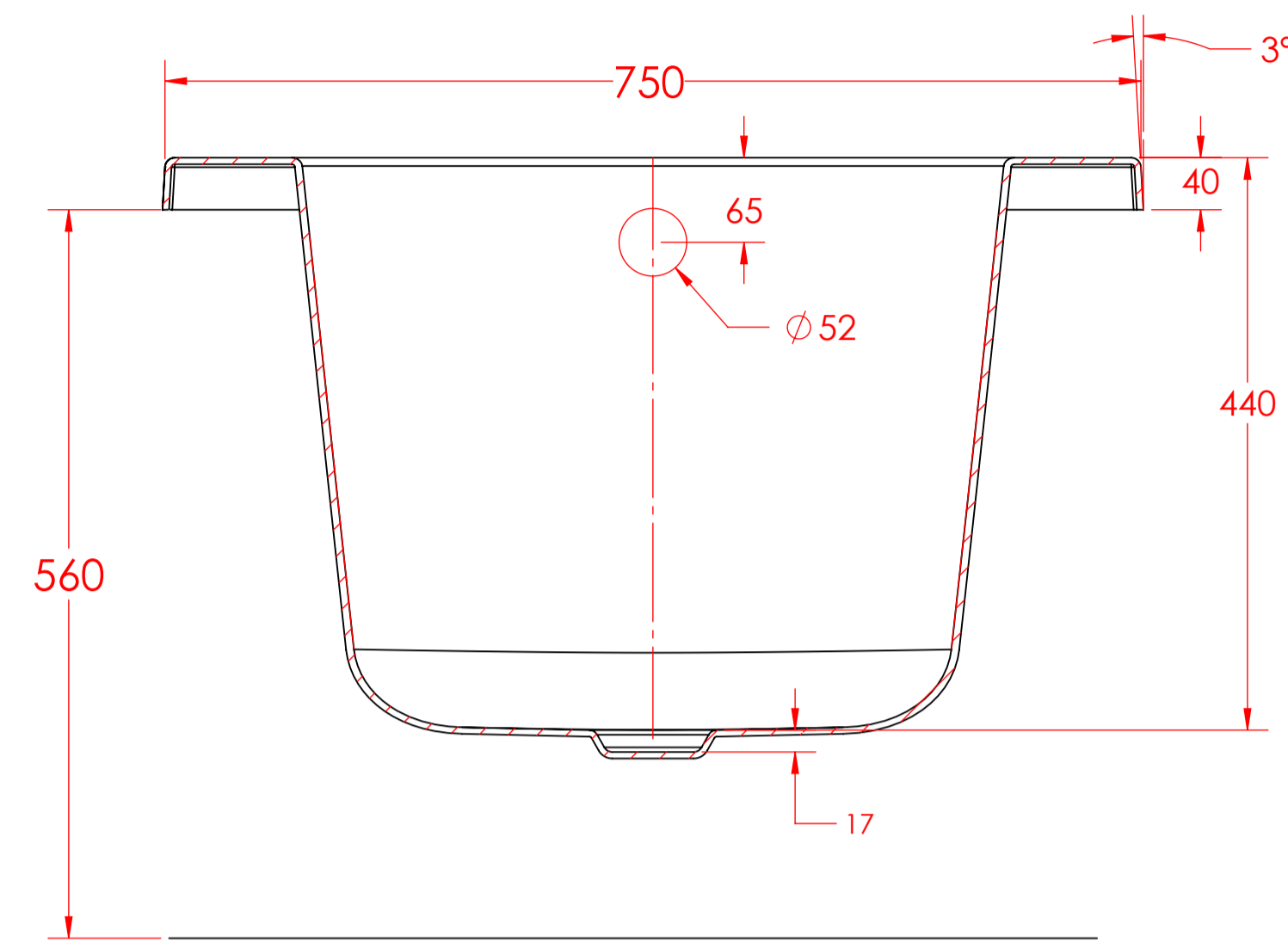
SECTION A-A
