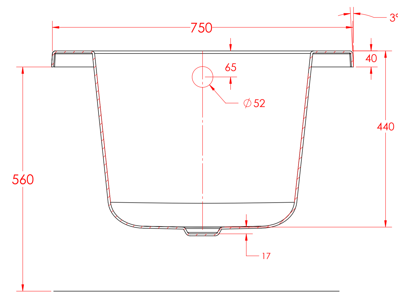
SECTION A-A
