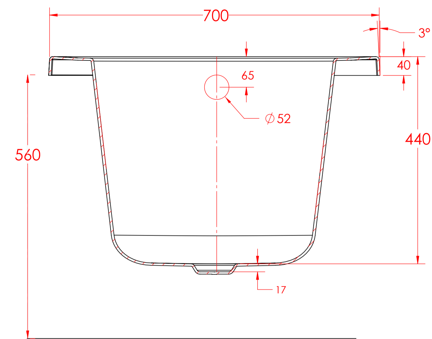
SECTION A-A
