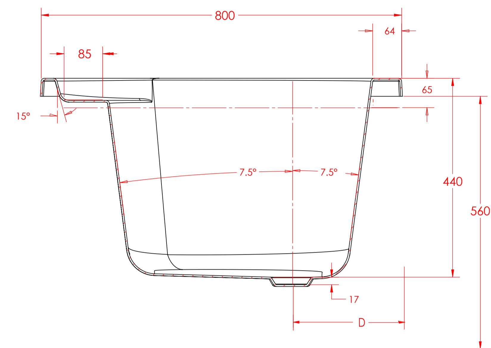
SECTION D-D SCALE 1 : 5
