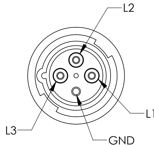
INPUT PLUG DETAIL IEC 60309 9H 100A / 3P4W
