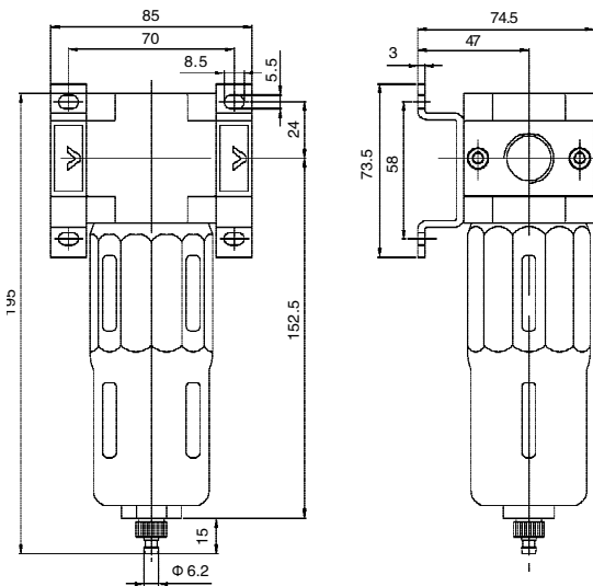
■ DF400-03、04、06
