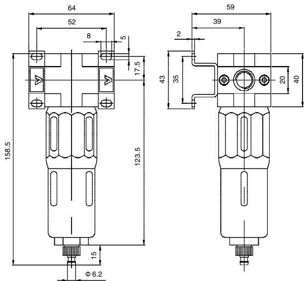
■ DF200-01、02、03
