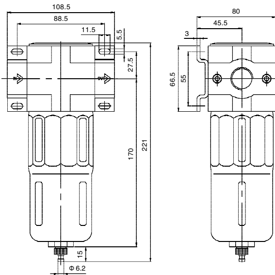
■ DF600-06、08
